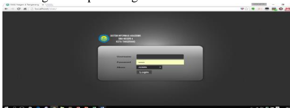
Gambar 5 Tampilan Login
