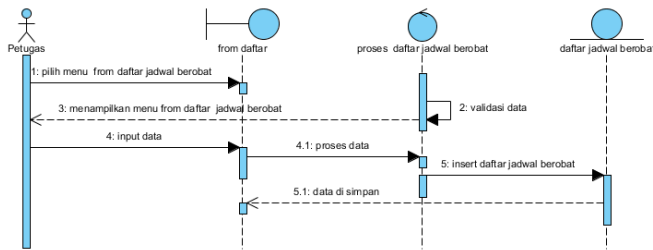
Gambar 19. Sequence Diagram Daftar Jadwal Berobat
