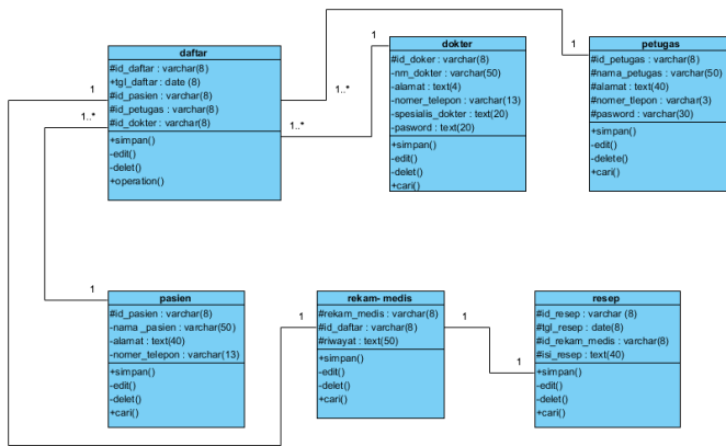
Gambar 20. Class Diagram yang diusulkan
