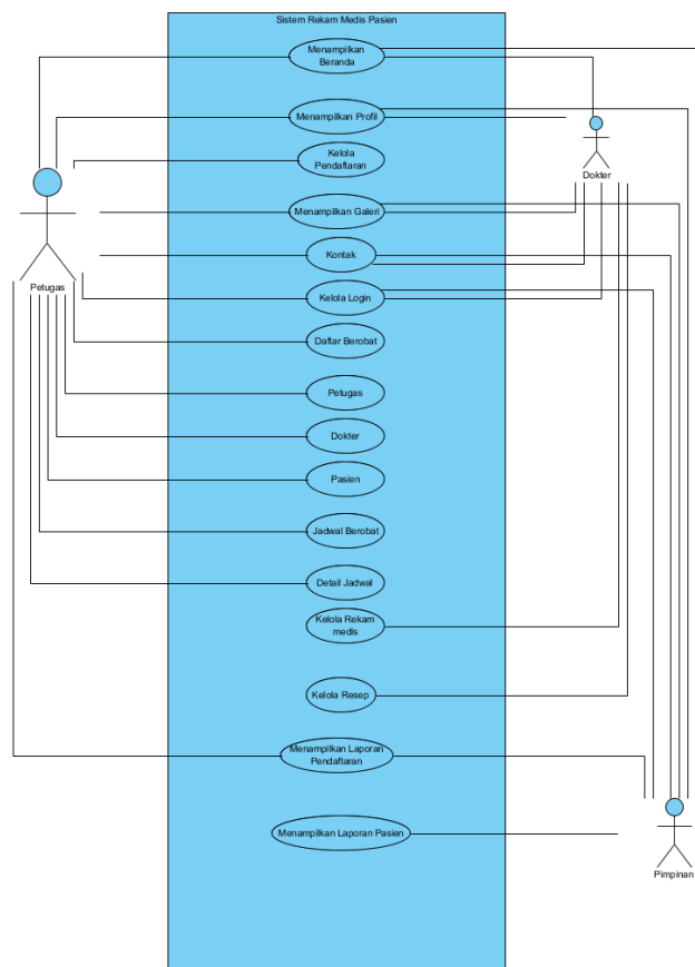
Gambar 4. Use Case Diagram yang diusulkan
