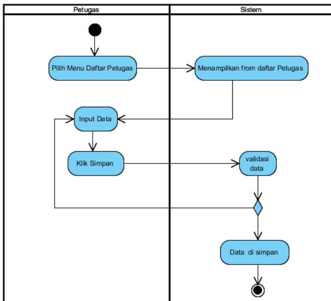
Gambar 11. Activity Diagram Daftar Petugas
